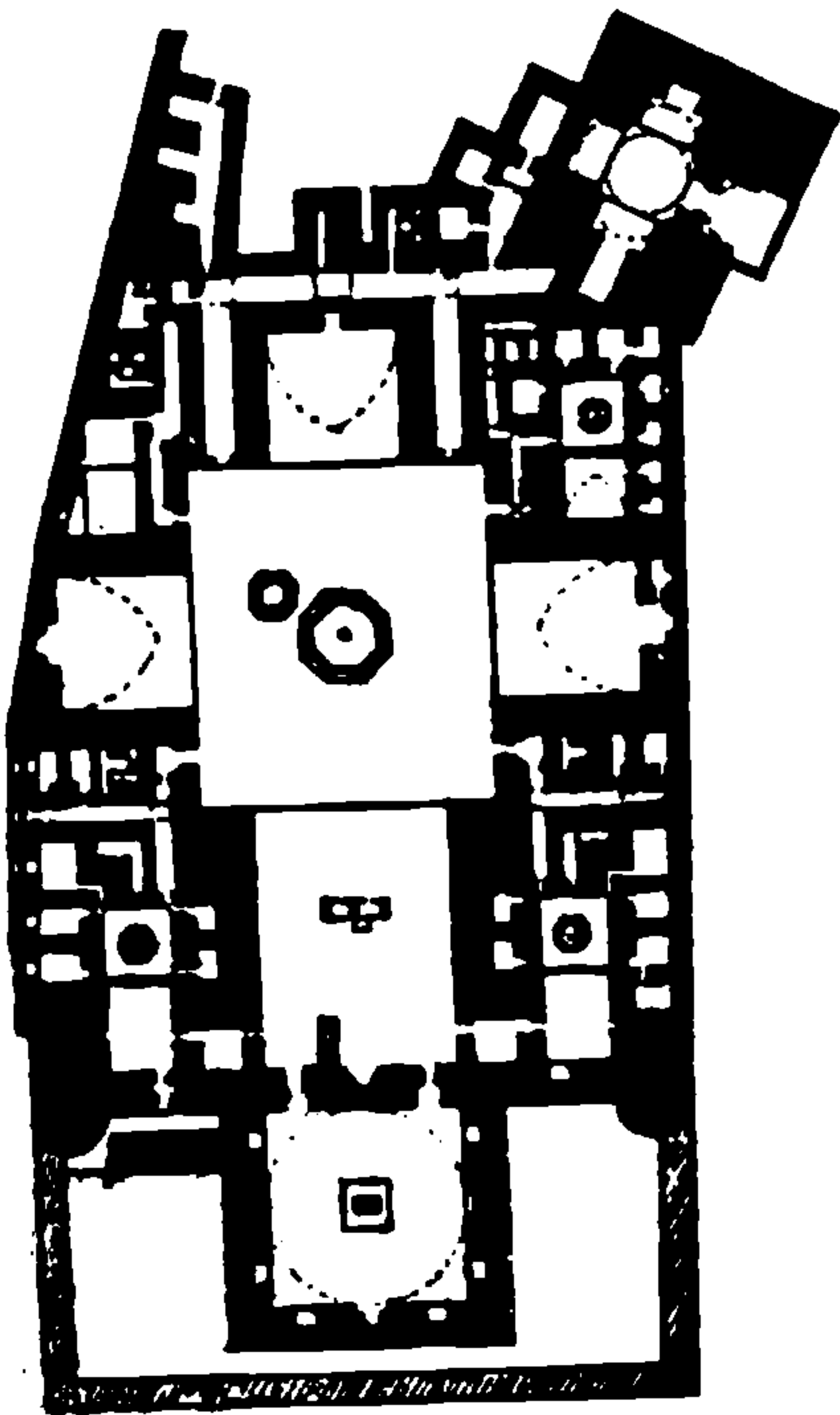
شکل ۶ - نقشه مدرسه سلطان حسن، قاهره
