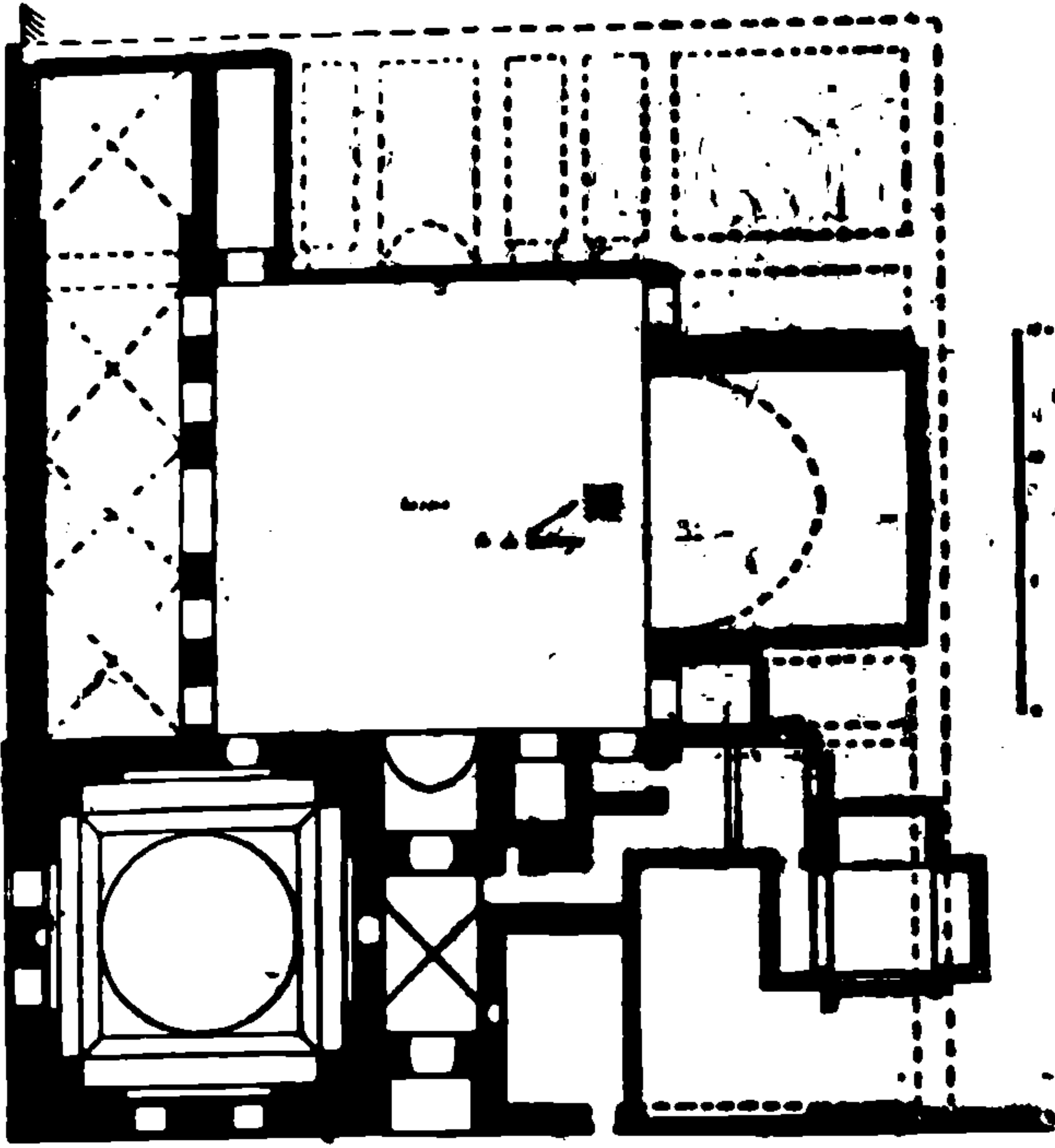
۹۔ دمشق : مدرسہ عادلہ (۸۹۱۹/۱۲۲۲ء)؛ قیہ دار عمارت، اوپر گنبد، الدر حجرہ نماز، اساتذہ و طلبہ کے رہائشی کمرے، ایک ایوان اور کمالوں سے مسقف ہال
