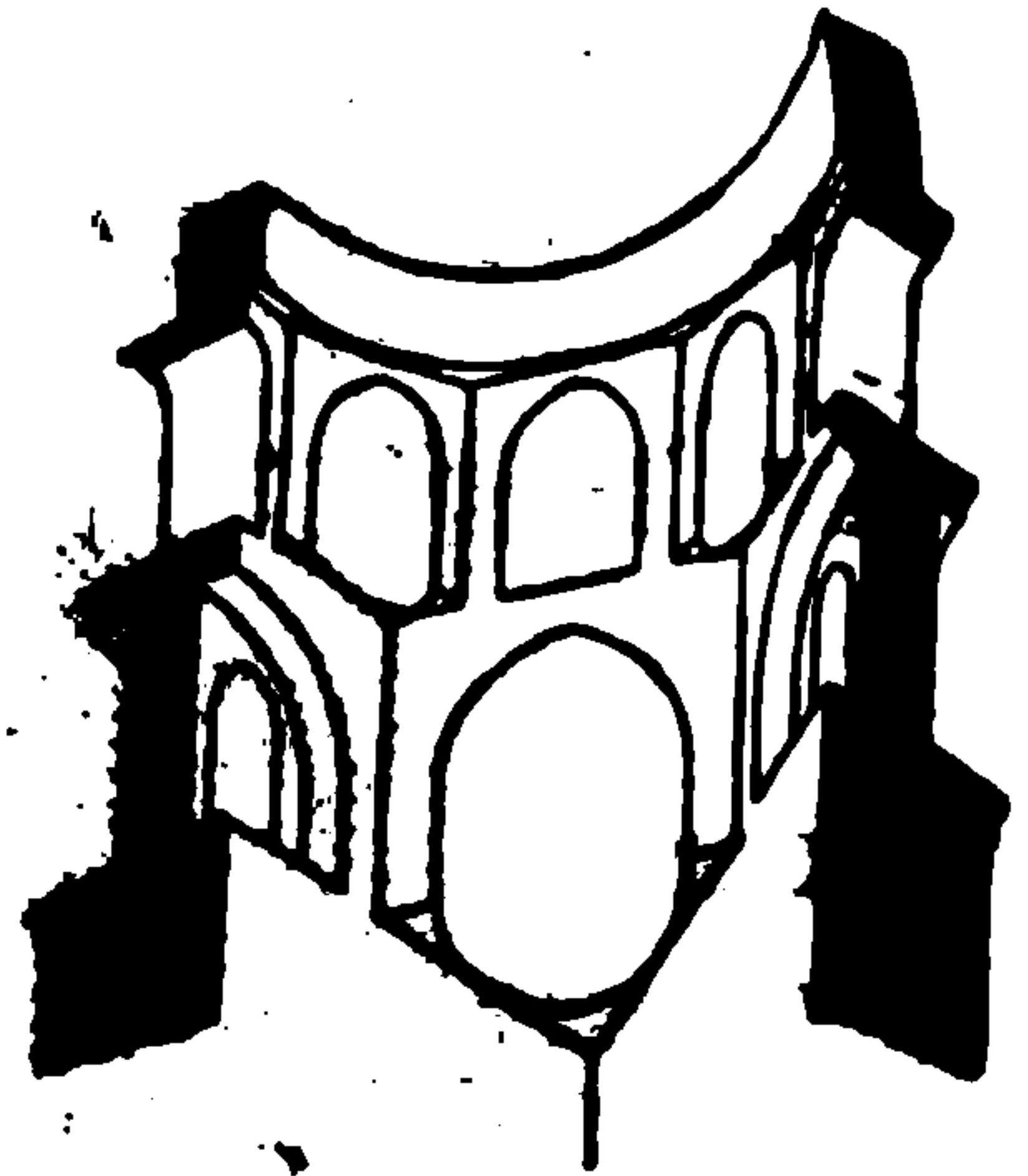
۱۲۔ ایروہ دیور میں لوہی کی تعمیر کی سکتی ہے مربع سے مدور تک پہنچنے کے لیے دو کثیرالزویا (آٹھ اور سولہ پہلو والے) منطوق سے گزرتے ہیں؛ اساس کا مکعب تو پتھر کا ہے، لیکن کثیرالزویا منطوق اور چھوٹے لچے اپنے کے ہیں
