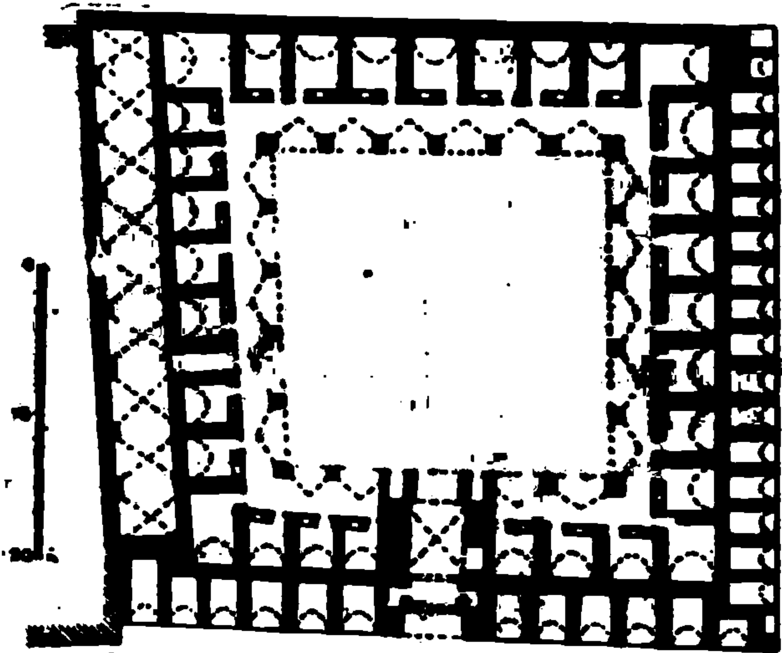
۱۹۔ حلب : خان النخاسین (دسویں / سولہویں صدی)؛ ہائے کا نقشہ۔ دکالیں بازار کا جز ہیں، خان کے دروازے کے معاذی واقع ہے۔ دکالیں صارت کے دائیں اور بائیں کی جانب ہیں۔ تاجروں کے گوداموں کے دروازے ایک حلام گردش میں ہیں، جس پر کمان چھت ہے اور جو سارے صحن کے اطراف چلی گئی ہے۔ پہلی منزل یعنی بالا خانے میں سکونت گاہیں کم و بیش زہریں منزل کے نقشے پر بنی ہیں
